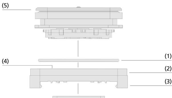
Systemaufbau Vakuum-Blocksauger Adapterplatten AP-S4
