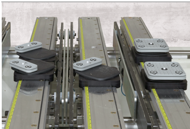
Adapter-Plates AP-S4 mit Blocksauger VCBL-B zum Aufspannen von unterschiedlichen Werkstückgeometrien
