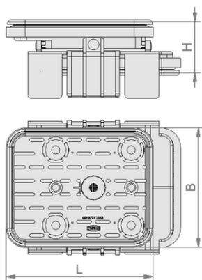
Konstruktionsdaten VCBL-K1 140x115x50
