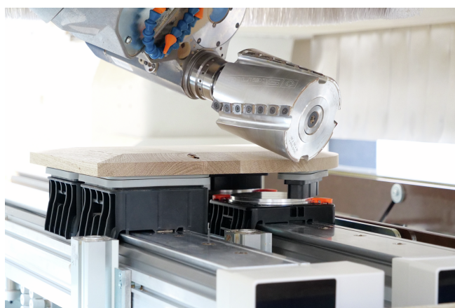
Blocksauger VCBL-S6 beim Einsatz auf SCM-Konsolen
