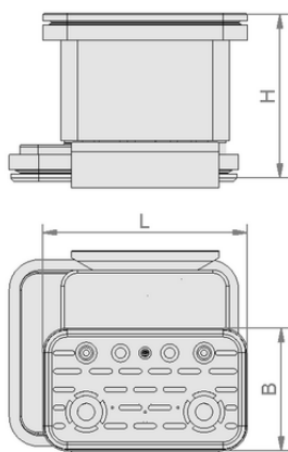
Konstruktionsdaten VCBL-K2 130x30x50 L
