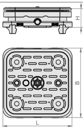
Konstruktionsdaten VCBL-S1 120x120x32.7 TV-S
