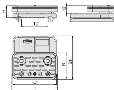
Konstruktionsdaten VCBL-S1 125x75x32.7 TV
