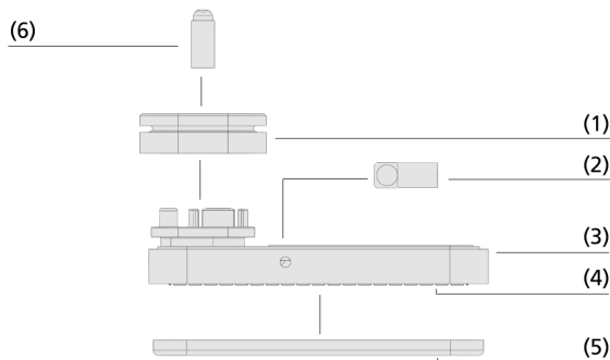
Systemaufbau Vakuum-Blocksauger VCBL-G-K1
