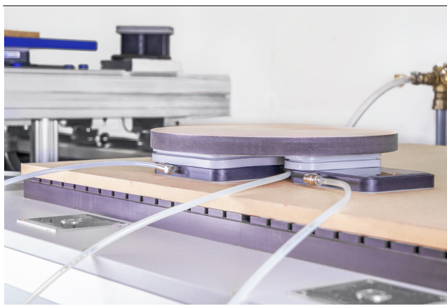
Blocksauger VCBL-G-K1 auf einer MDF-Verschleißplatte
