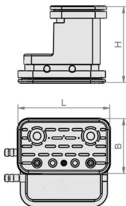
Konstruktionsdaten VCBL-G-K2 120x50x100 ST
