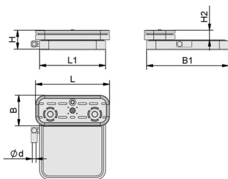
Konstruktionsdaten VCBL-G-K1 120x50x30
