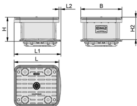
Konstruktionsdaten VCBL-B 140x130x74 TV
