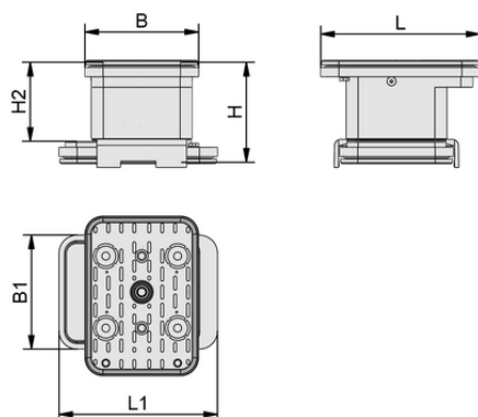
Konstruktionsdaten VCBL-K2-PRO 160x115x100 Q
