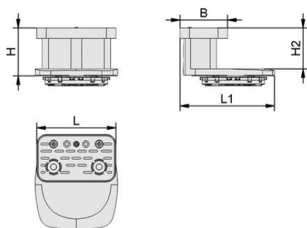
Konstruktionsdaten VCBL-B 120x50x48 TV
