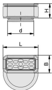
Konstruktionsdaten ISCUP Cup 2 80x40x30
