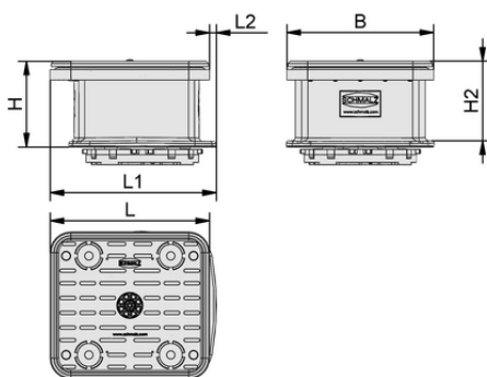
Konstruktionsdaten VCBL-B 140x130x48 TV
