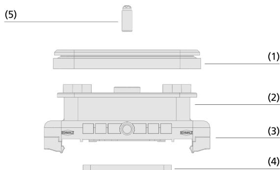
Systemaufbau Vakuum-Blocksauger VCBL-S4
