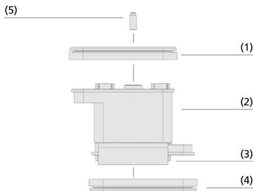
Systemaufbau Vakuum-Blocksauger VCBL-K2
