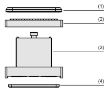
Systemaufbau Vakuum-Blocksauger VCBL-K2-HD
