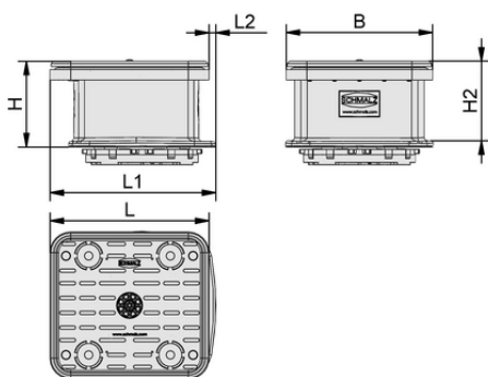
Konstruktionsdaten VCBL-B 140x130x29 TV
