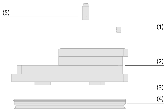
Systemaufbau Vakuum-Blocksauger VCBL-R 50
