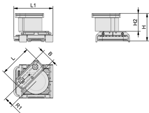
Konstruktionsdaten VCBL-K2 120x50x100 D-360
