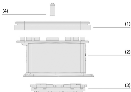
Systemaufbau Vakuum-Blocksauger VCBL-B
