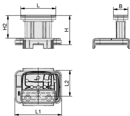
Konstruktionsdaten VCBL-K1-PRO 125x75x100 L
