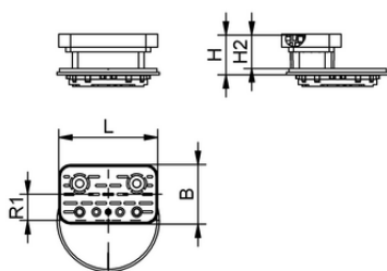
Konstruktionsdaten VCBL-S6-CUP 125x75x85 TV+ME
