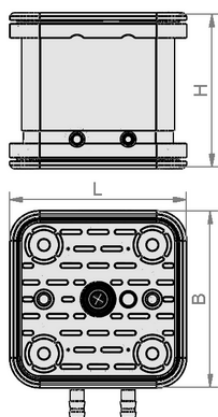
Konstruktionsdaten VCBL-G-K2 120x120x100 ST+AS
