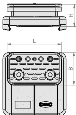
Konstruktionsdaten VCBL-S4 120x50x50 TV
