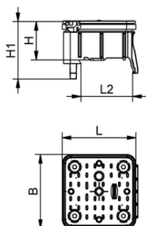
Konstruktionsdaten VCBL-S6 145x145x110 TV+ME
