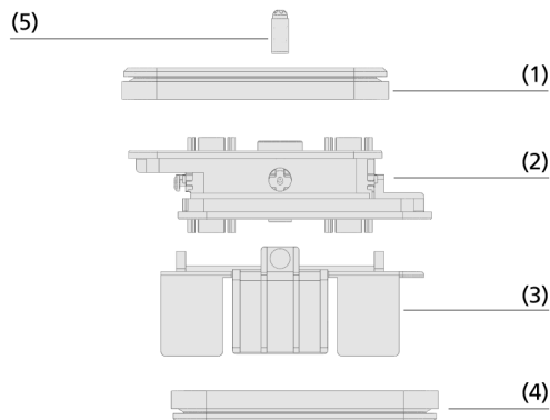
Systemaufbau Vakuum-Blocksauger VCBL-K1
