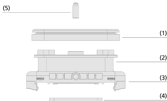
Systemaufbau Vakuum-Blocksauger VCBL-S1
