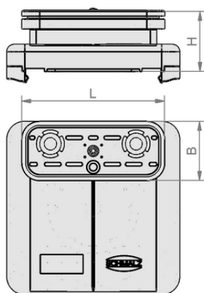
Konstruktionsdaten VCBL-S1 125x75x32.7 TV-S
