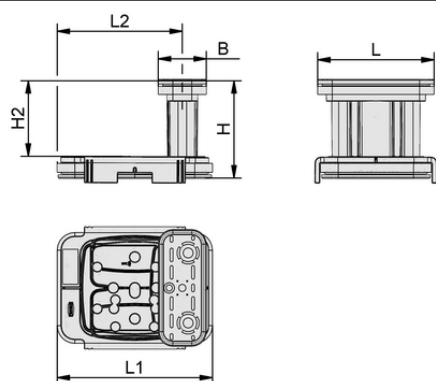
Konstruktionsdaten VCBL-K2-PRO 120x50x100 Q
