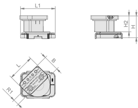
Konstruktionsdaten VCBL-K1-PRO 120x50x100 D-360
