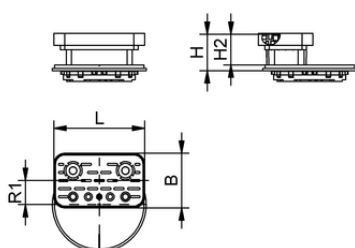
Konstruktionsdaten VCBL-S6-CUP 130x30x85 TV
