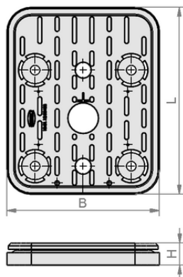
Konstruktionsdaten VCSP-O 140x115x16.5 TPE
